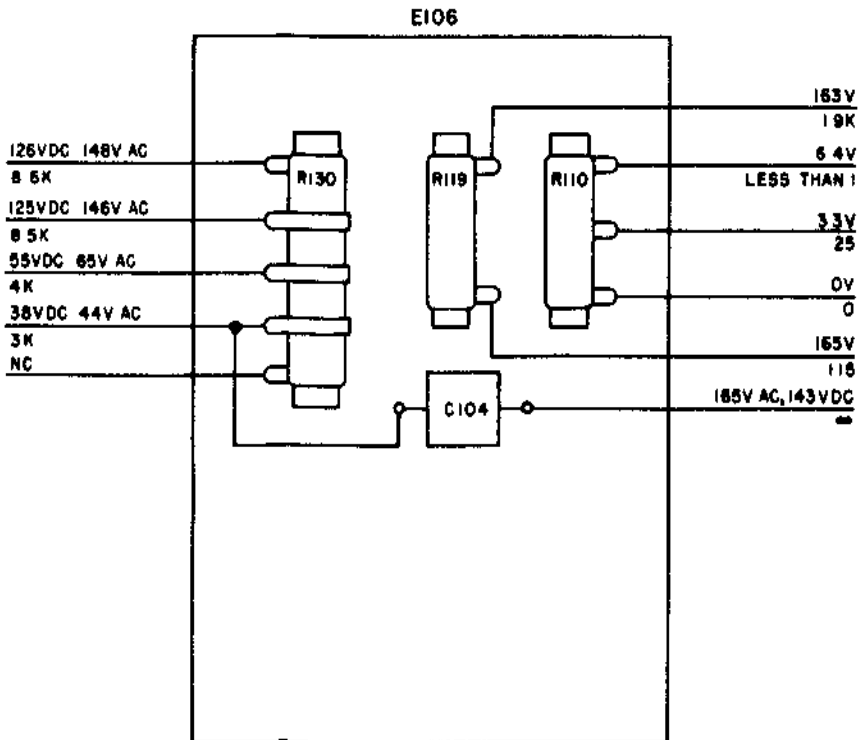
D TV-7B/U
