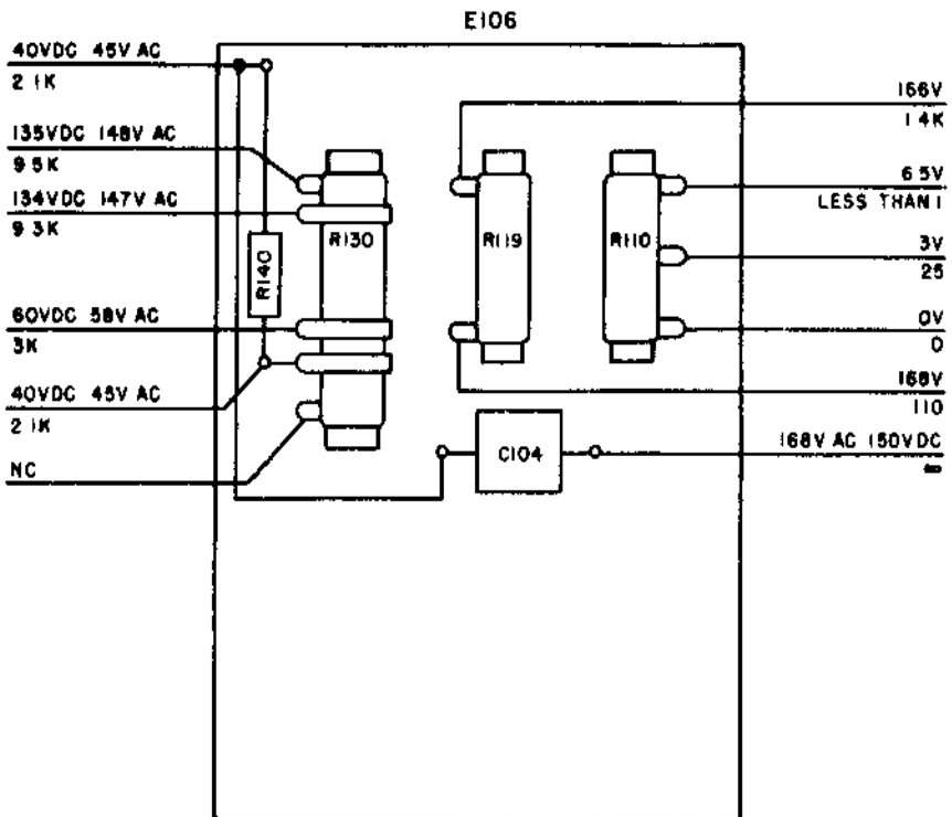
E TV-7D/U
